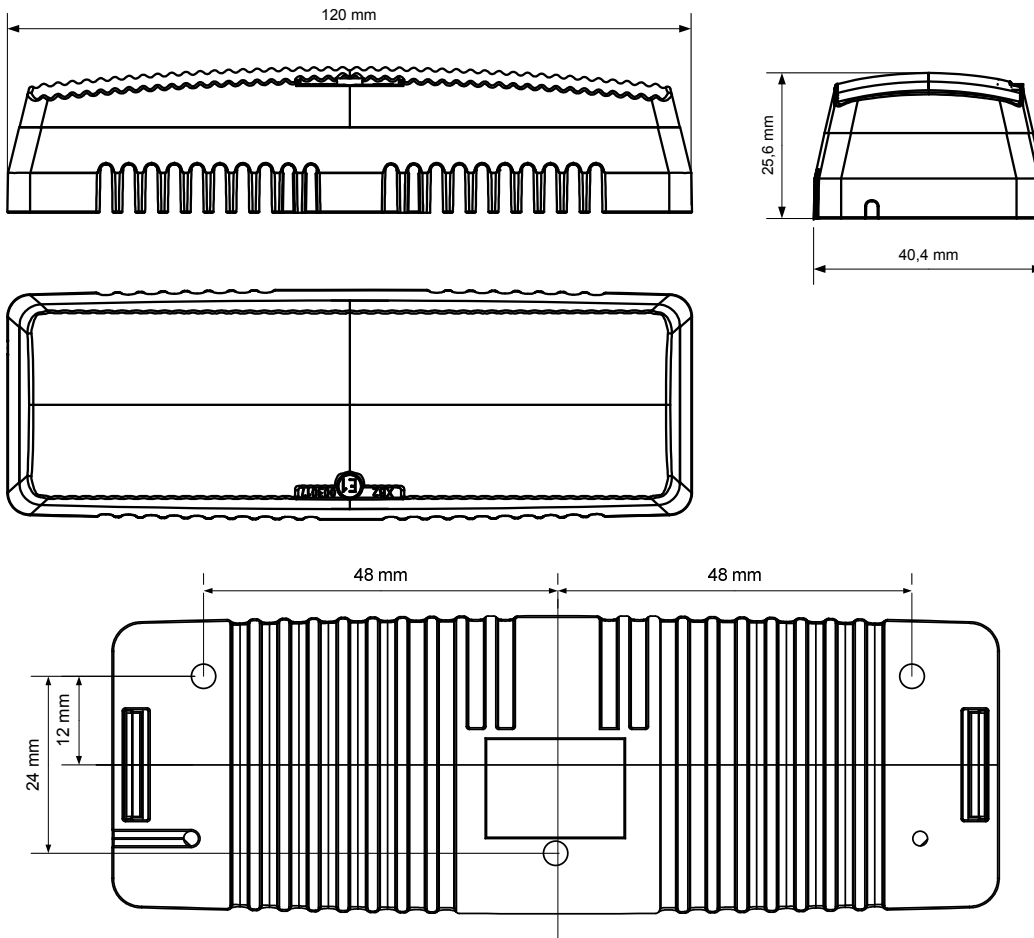
Maßzeichnung
